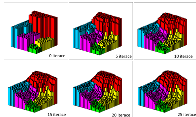
Pycnophylactická interpolace
