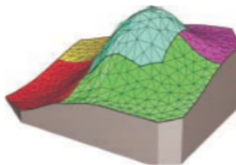
Shlazený TIN
